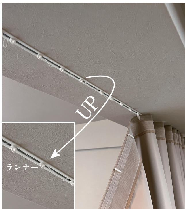
レール工事（下地序盤にバッチリ施工！）
