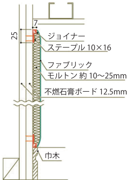
ファブエースソフトタイプ断面図
